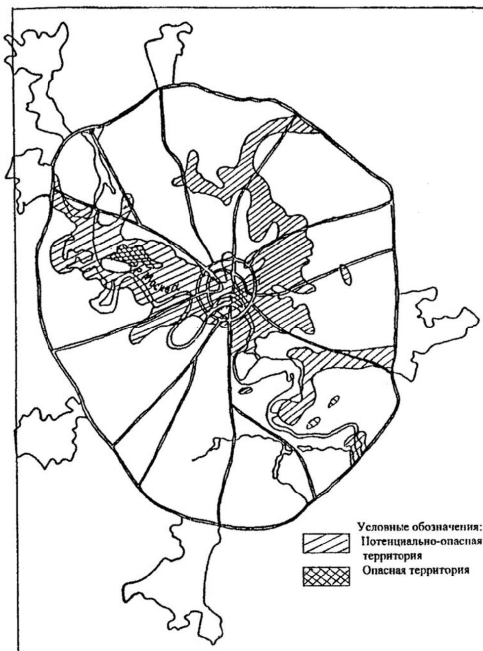
Схематическая карта инженерно-геологического районирования центральной части Москвы по геологическому строению и условиям взаимосвязи водоносных
